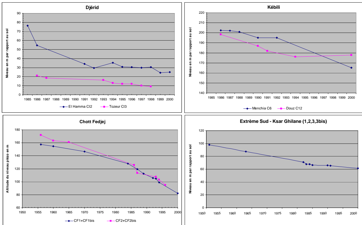
Figure n° 36 - Continental Intercalaire - Exemples de rabattement en Tunisie
