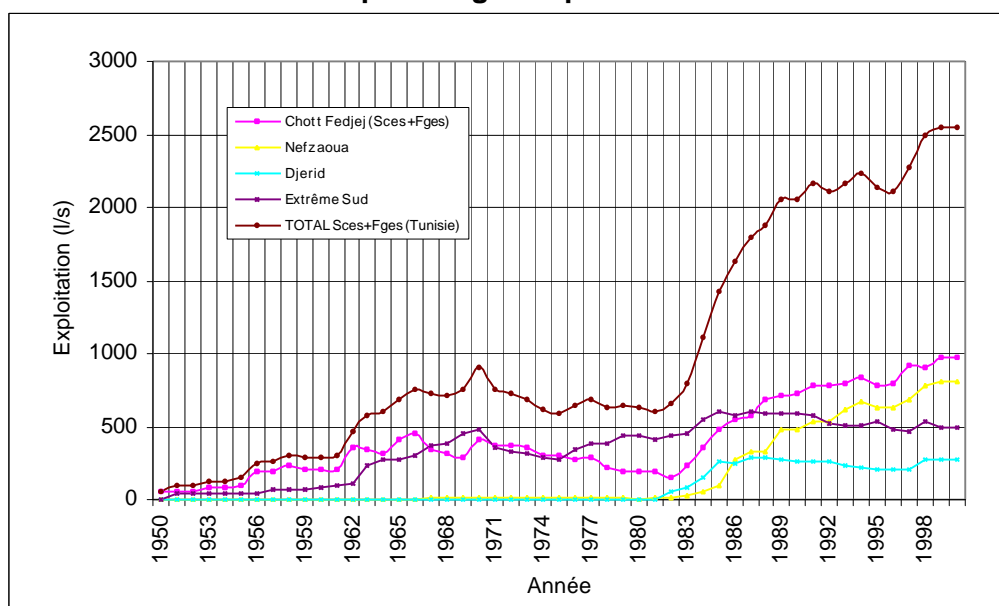
Figure n° 31 - Exploitation du Continental Intercalaire en Tunisie par forages et par sources en l/s
