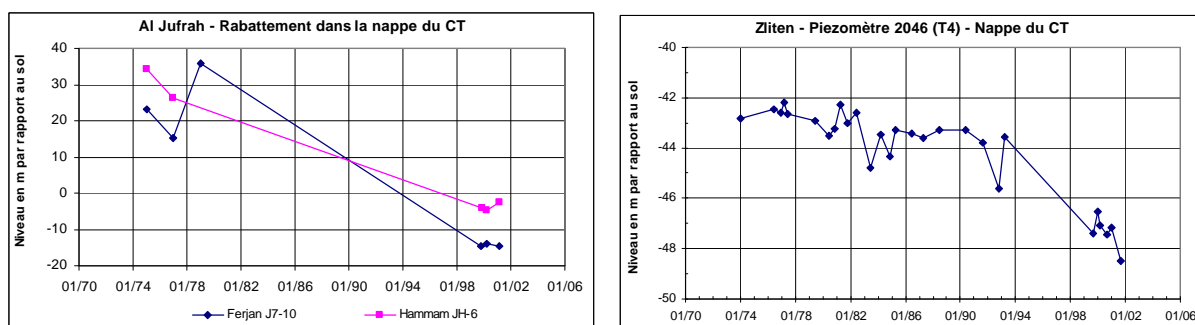
Figure n° 34 - Complexe Terminal - Exemples de rabattement en Libye
