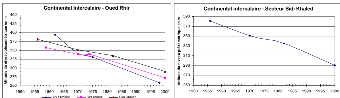
Figure n° 35 - Continental Intercalaire - Exemples de rabattements en Algérie
