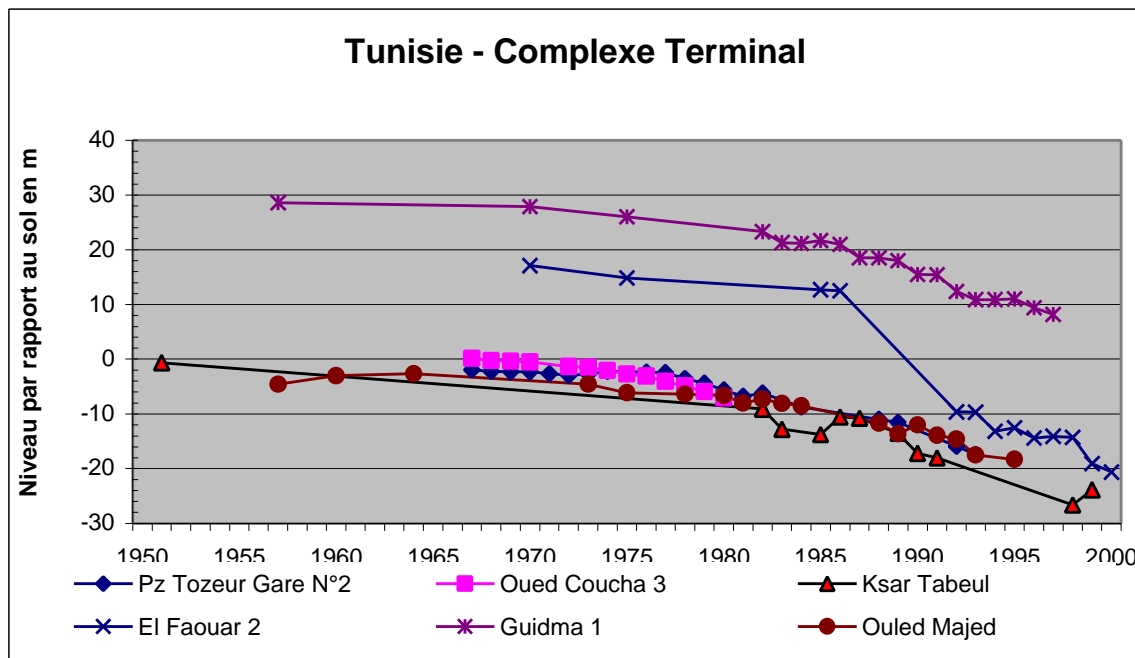
Figure n° 33 - Complexe Terminal - Exemples de rabattements en Tunisie
