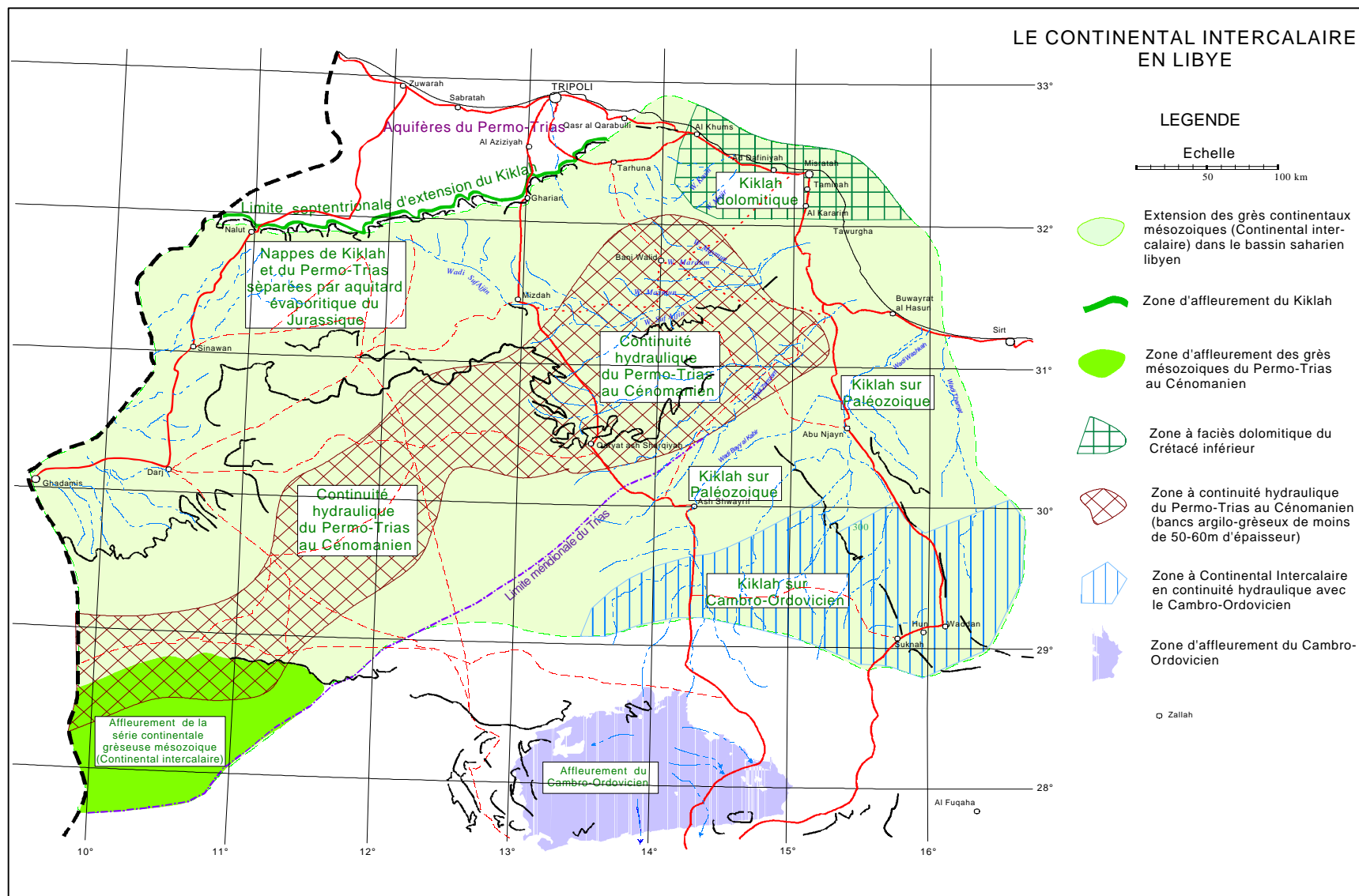
Figure n°12 - Composition du Continental intercalaire en Libye
