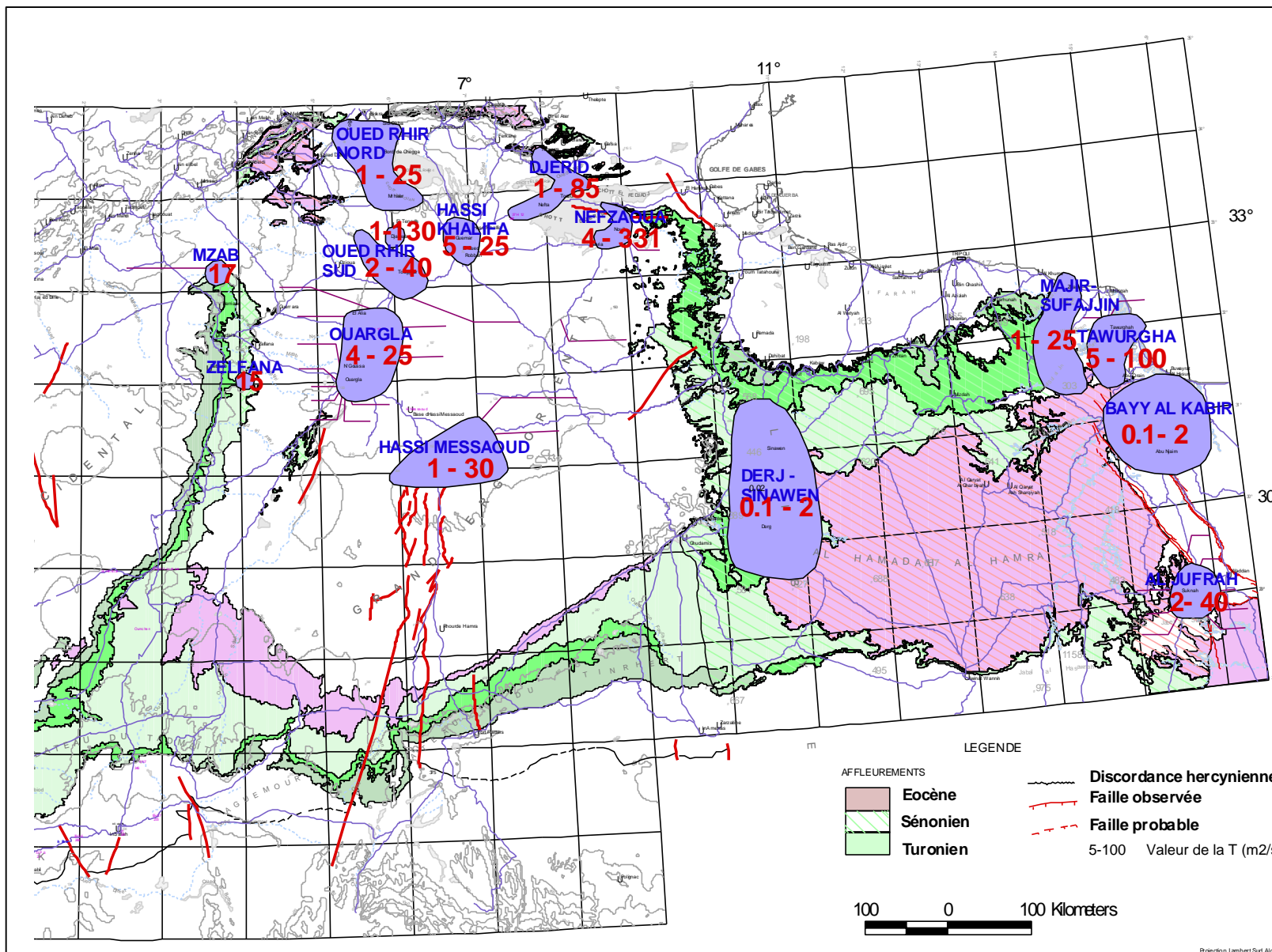
Figure n° 28 : Carte de transmissivités du Complexe terminal
