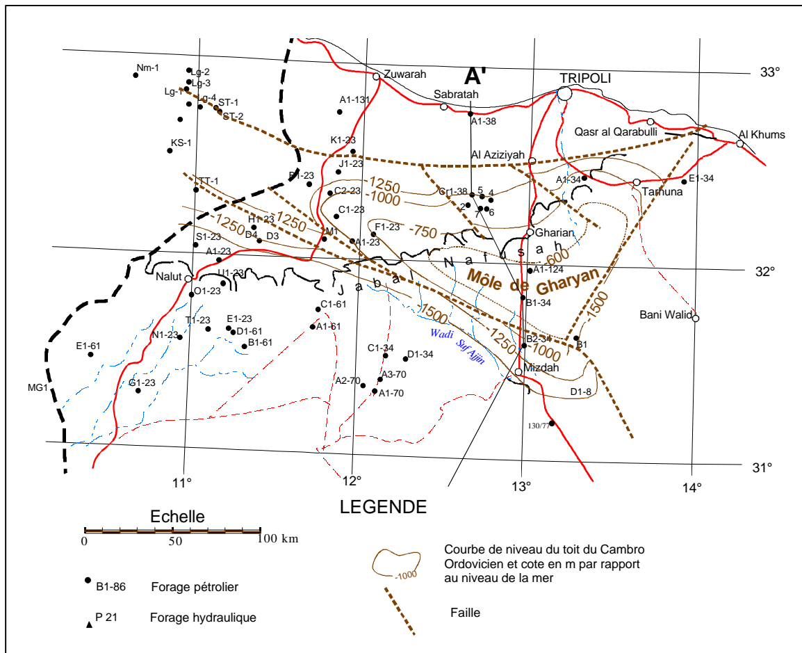
Figure n°16 : Liaison avec la plaine de la Jifarah
