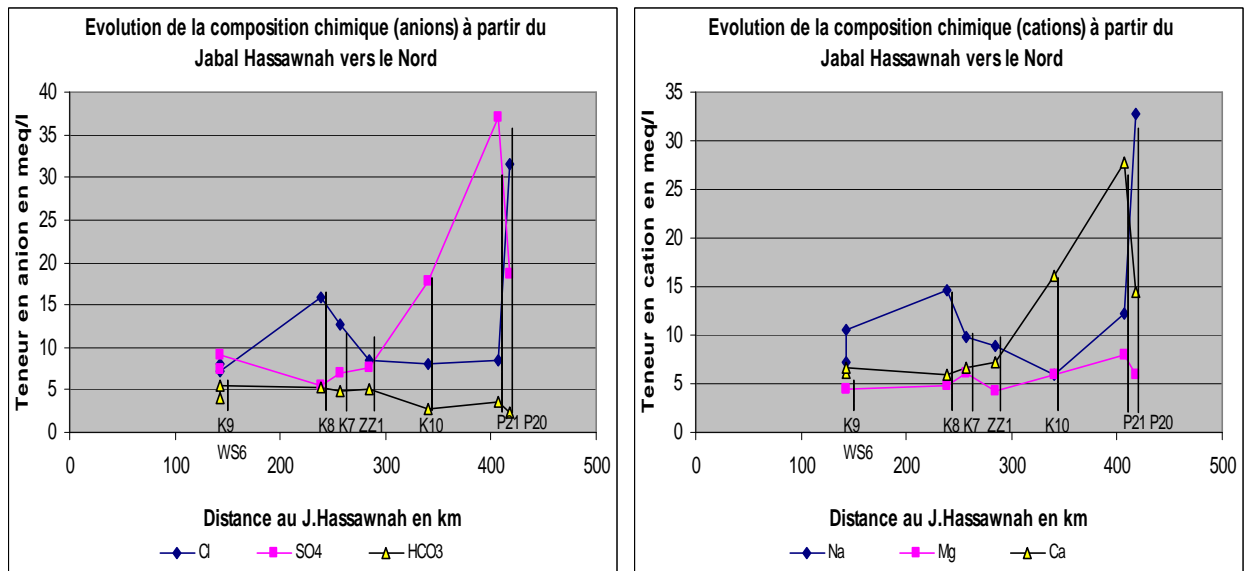
Figure n° 43 – Evolution de la composition chimique des eaux du Continental Intercalaire en Libye depuis Jabal hassawna vers le Nord
