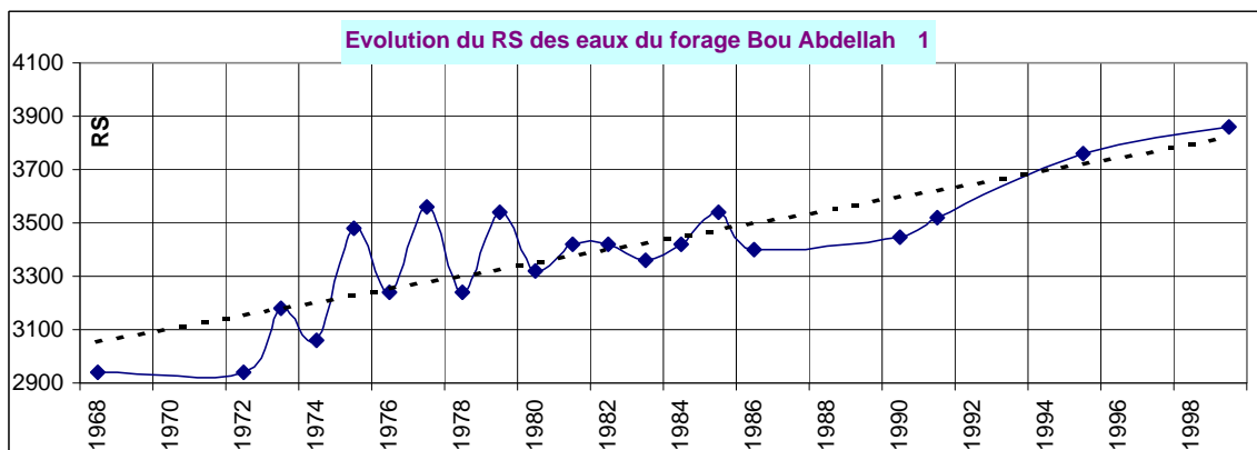
Figure n°38 : Evolution de la salinité de l'eau du Complexe Terminal dans la Presqu'île de Kébili (Nefzaoua-Tunisie)
