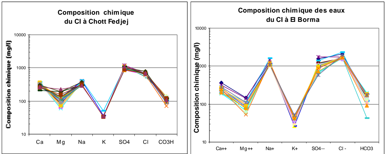
Figure n° 42 - Composition chimique des eaux du Continental Intercalaire en Tunisie
