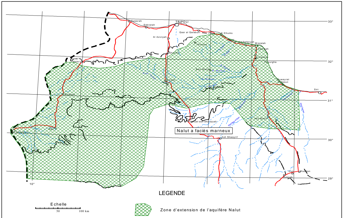
Figure n°9 - Extension de l'aquifère Nalut (Cénomano-Turonien) en Libye
