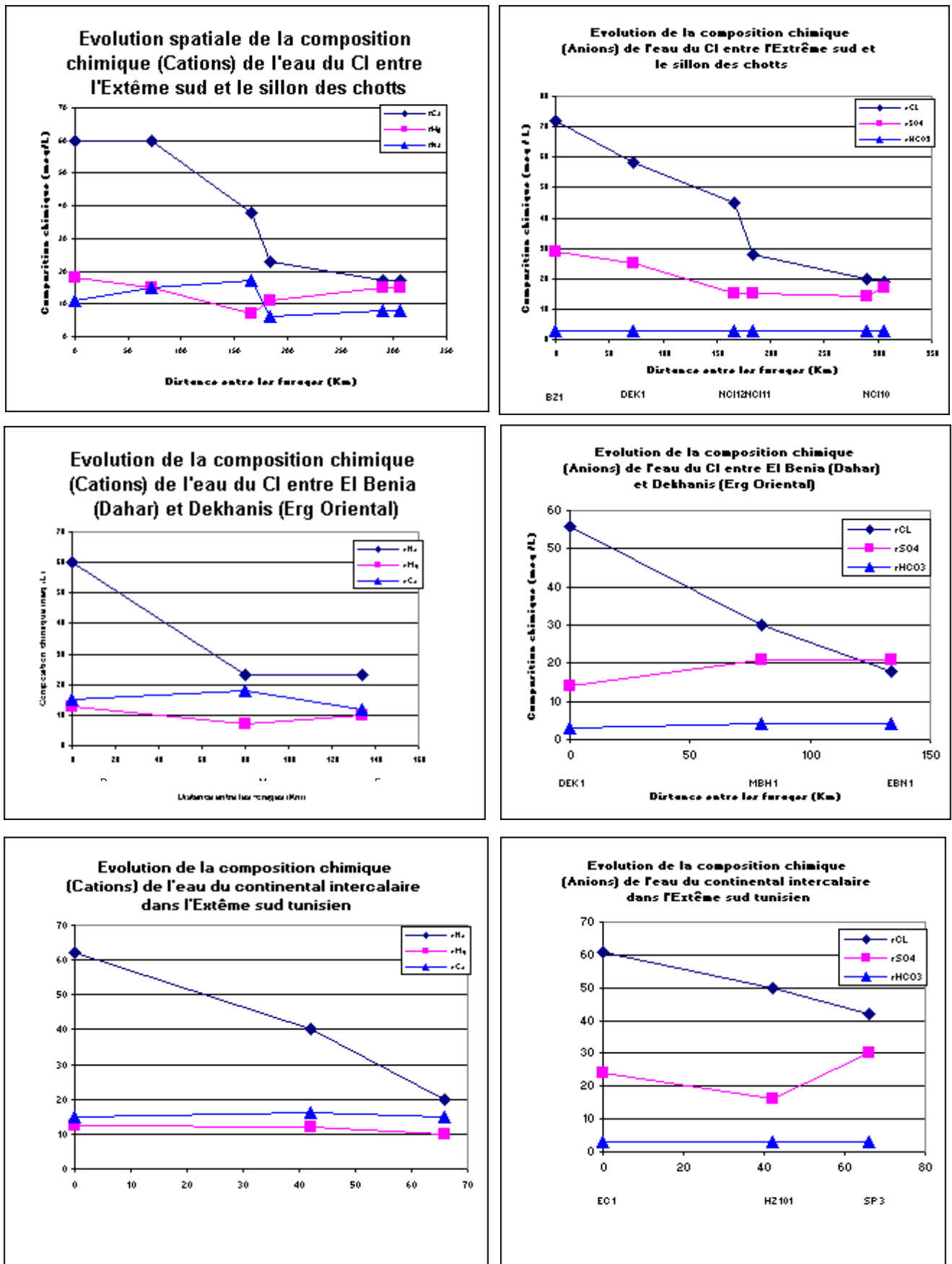
Figure n° 41 - Evolution de la composition chimique des eaux du CI en fonction de l'éloignement de la zone de recharge (Tunisie)
