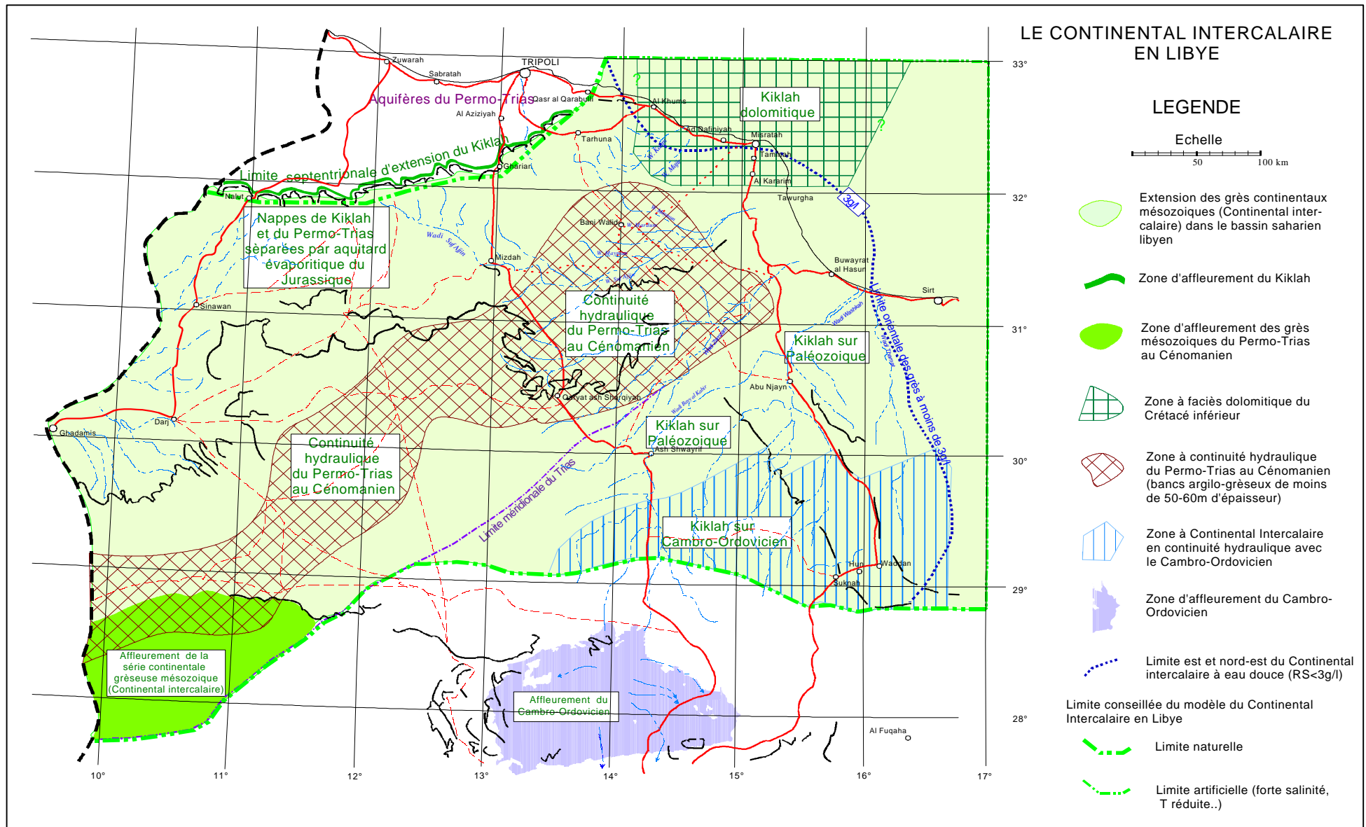
Figure n°23 - Limite conseillée pour la couche du modèle représentant le Continental Intercalaire
