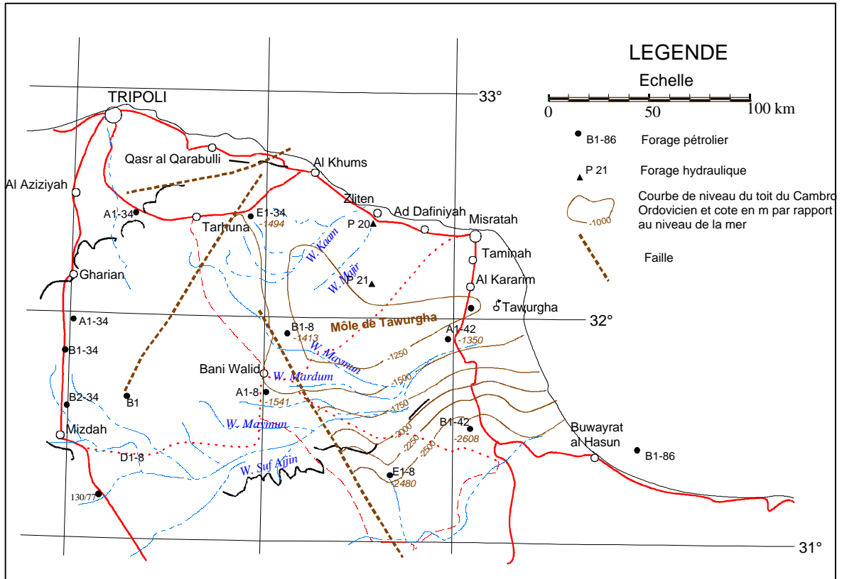
Figure n°19 : Toit du Cambro-Ordovicien autour de la source de Tawurgha
