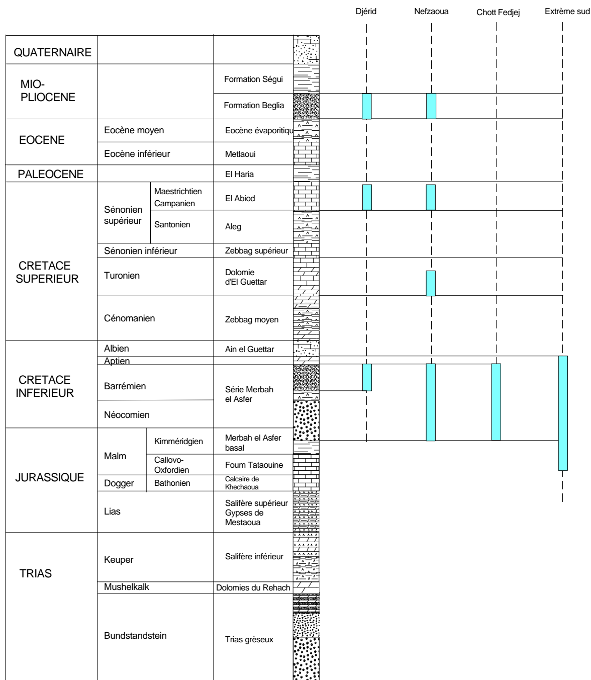
Figure n°8 - Les formations géologiques et les aquifères du sud tunisien
