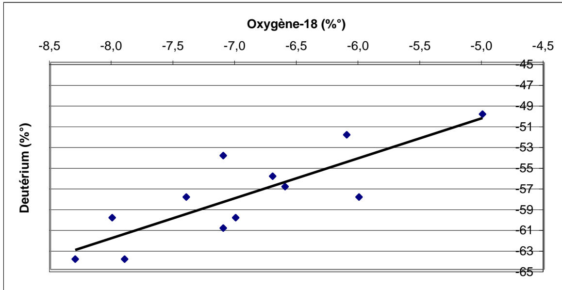
Figure n°45: Corrélation oxygène-18/deuterium des eaux du CI du bassin du Grand Erg Occidental (Algérie)
