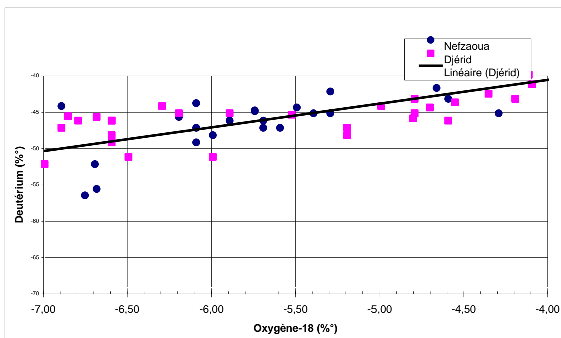
Figure n°48: Composition isotopique de l'eau du CT dans le Sud tunisien
