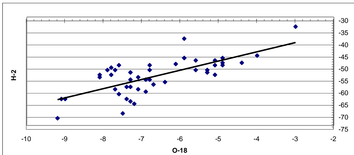
Figure n°47: Composition isotopique des eaux du CT en Algérie
