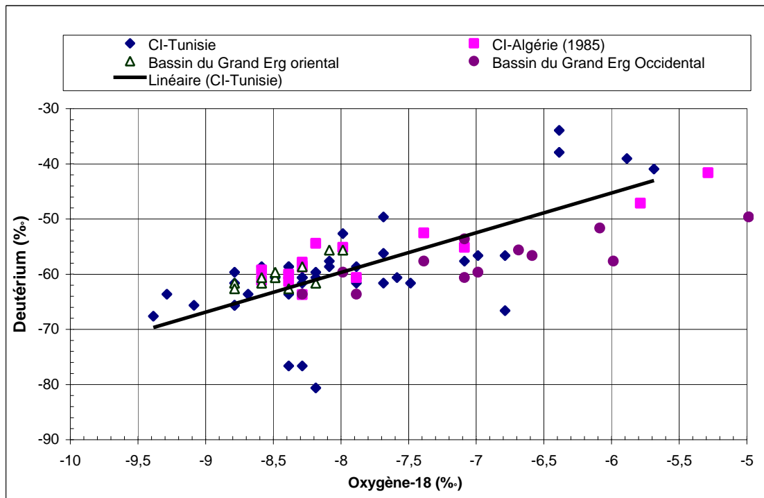
Figure n°44:Composition isotopique des eaux du Continental intercalaire en Algérie et en Tunisie
