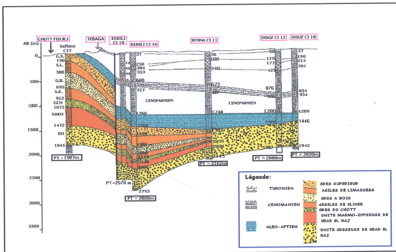
Figure n°15 : Corrélation Nord-Sud à travers la Nefzaoua entre Seftimi (Chott Fedjej) et Douz (Nefzaoua).
