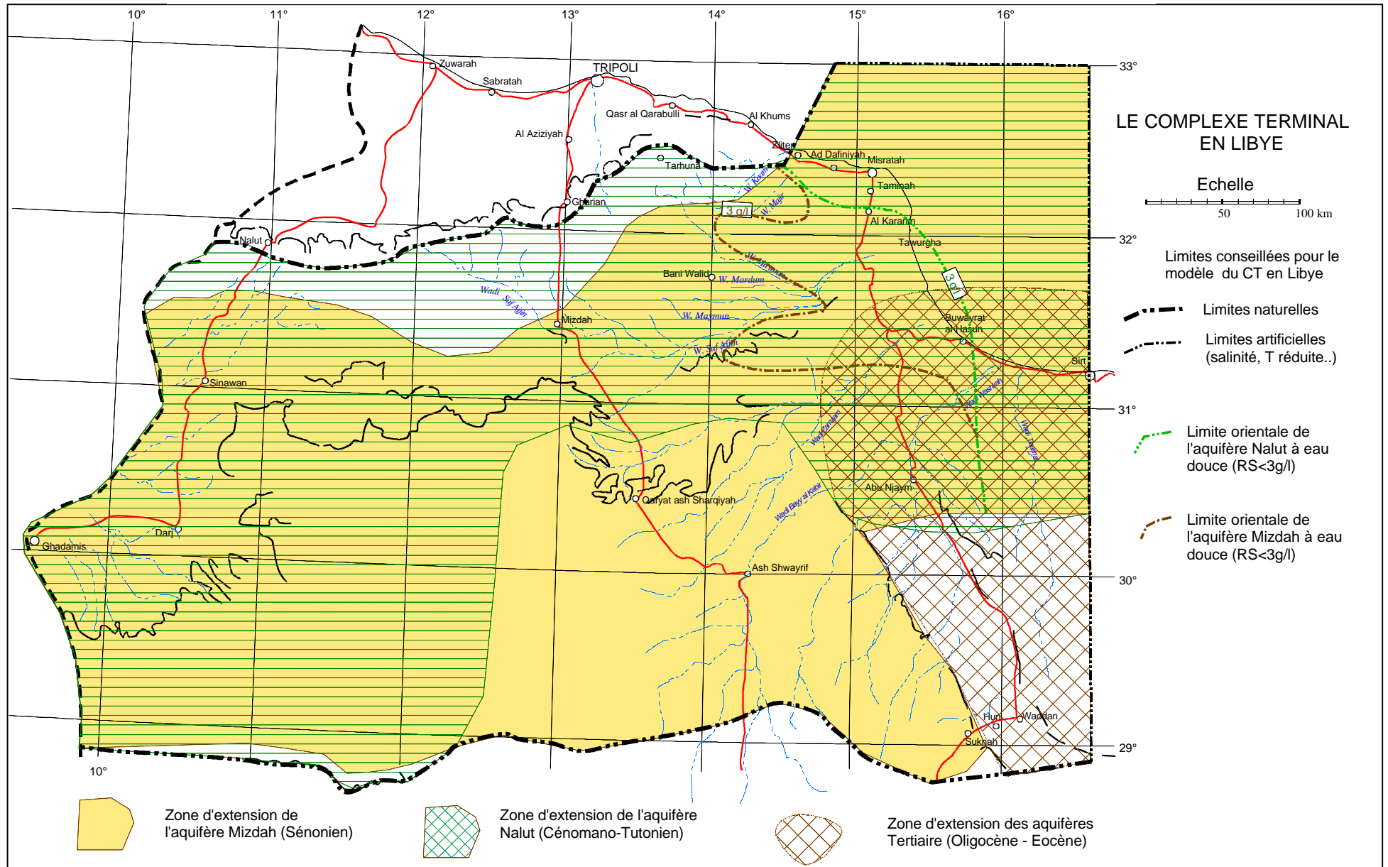
Figure n°22 - Limite conseillée pour la couche représentant le Complexe Terminal
