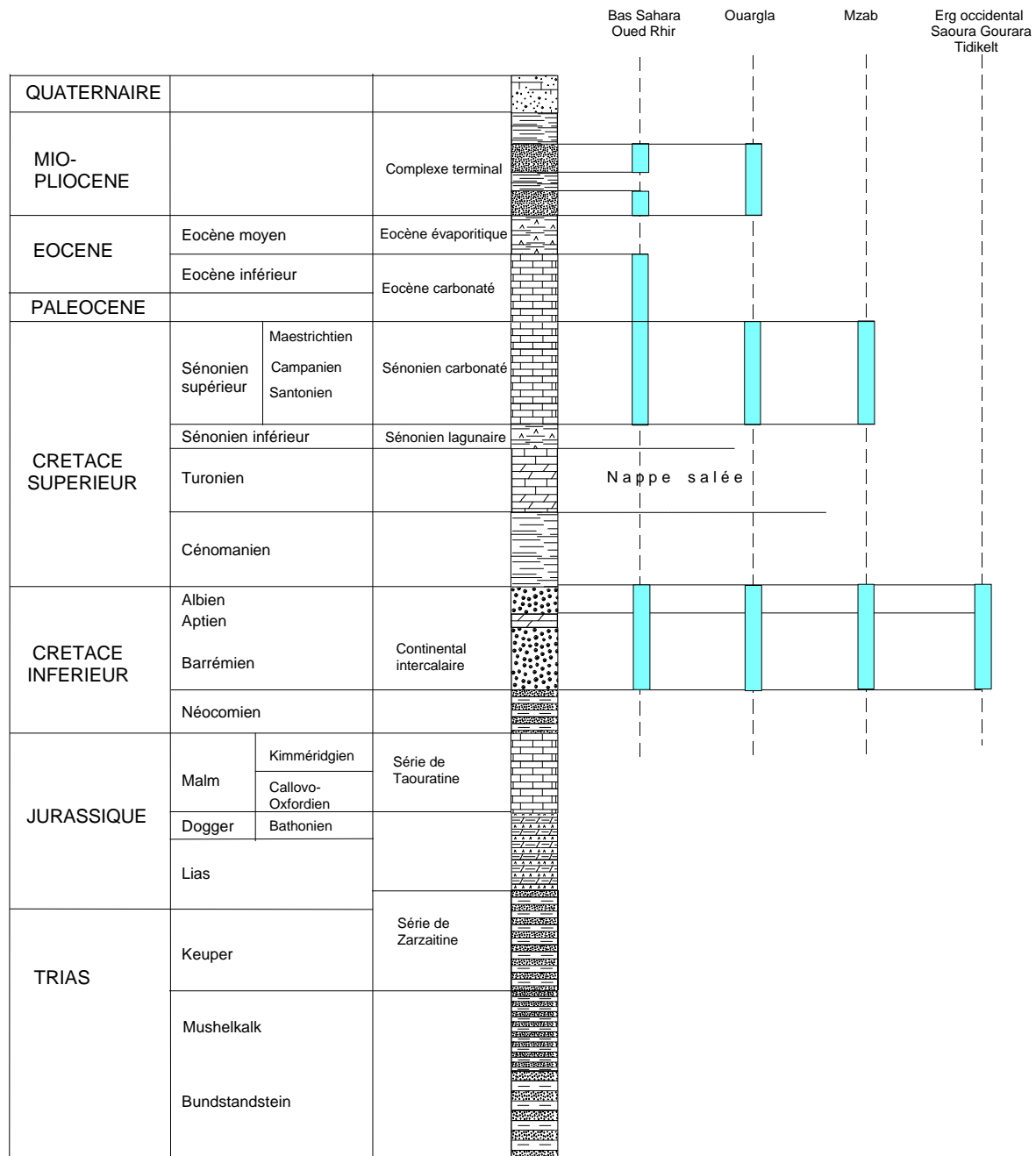
Figure n°6 - Les formations géologiques et les aquifères du bassin saharien algérien
