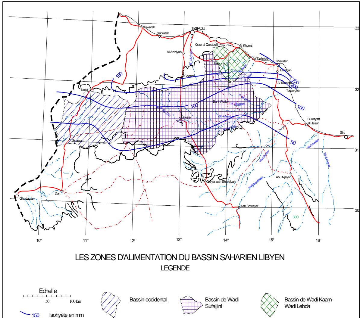
Figure 24 - Les zones d'alimentation des nappes du Crétacé supérieur en Libye
