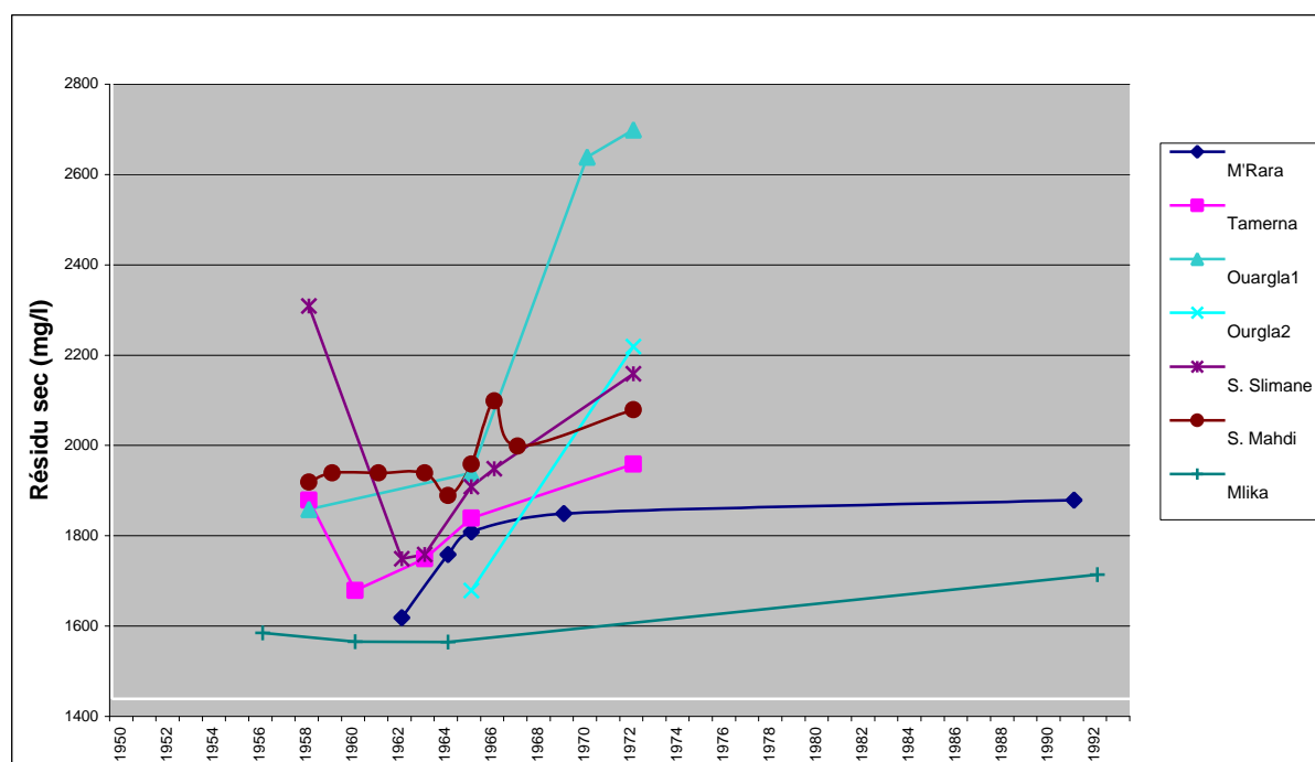
Figure n°40: Exemples de tendance à l'accroissement de la salinité du Cl en Algérie
