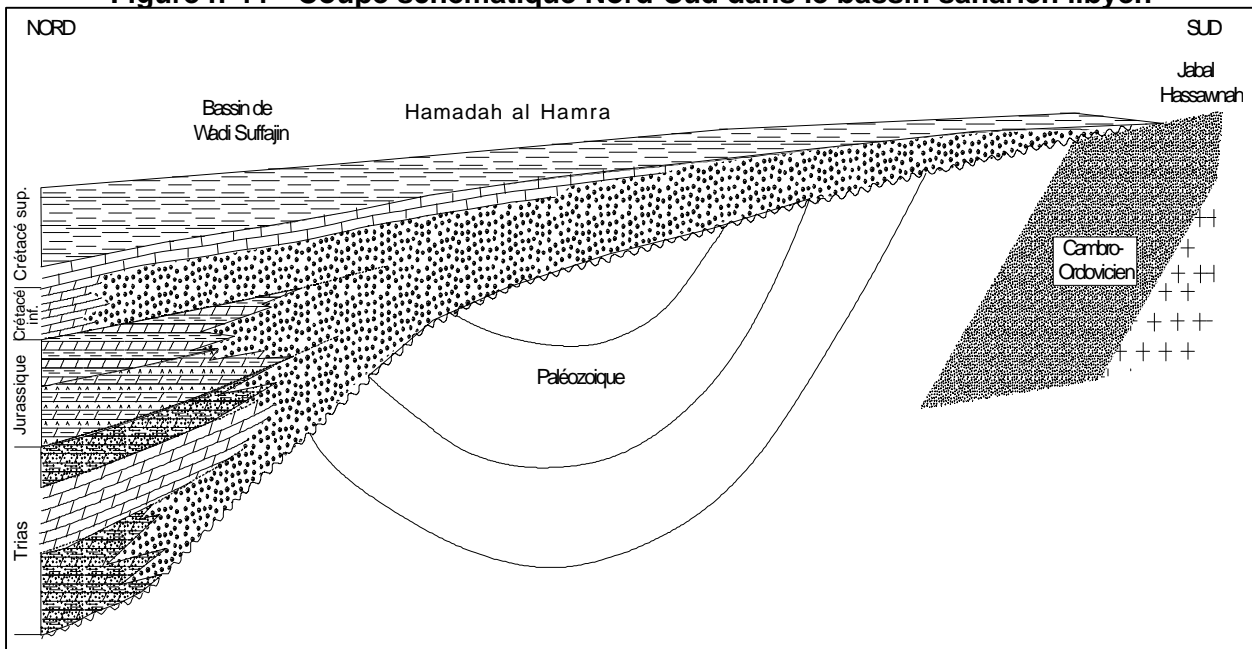
Figure n°11 - Coupe schématique Nord-Sud dans le bassin saharien libyen
