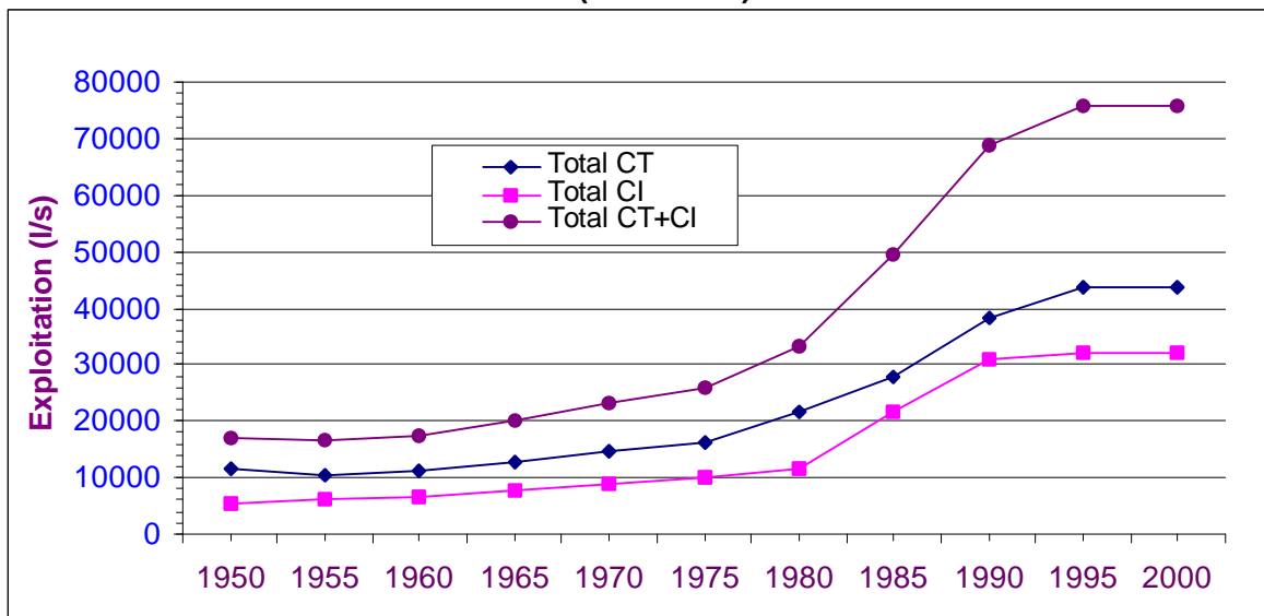
Figure n° 30 - Prélèvements globaux sur le CI et le CT dans les trois pays en l/s (1950-2000)
