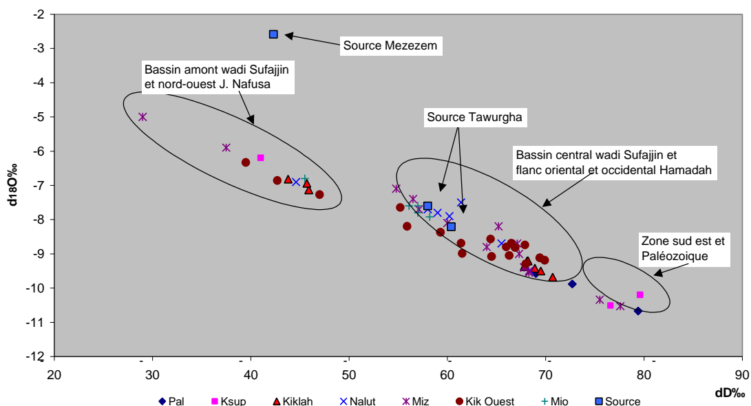
Figure n°46 : Composition en isotopes stables des eaux d'El Hamada El Hamra en Libye
