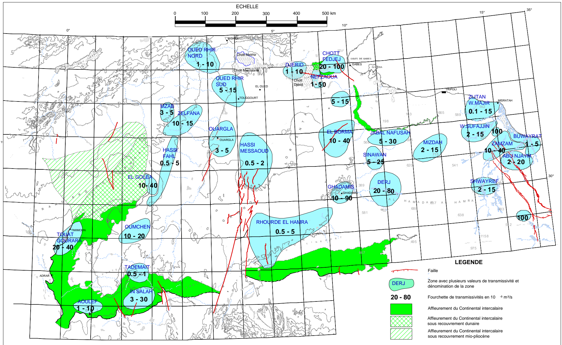
Figure n° 29 - Carte des transmissivités du Continental Intercalaire Tunisie
